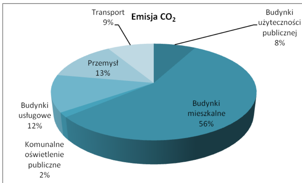
Rysunek 16. Procentowy udział sektorów w emisji CO 2
